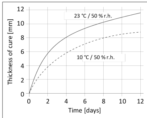
Diagrama 1: Velocidad de curado para Sikaflex® Fix
