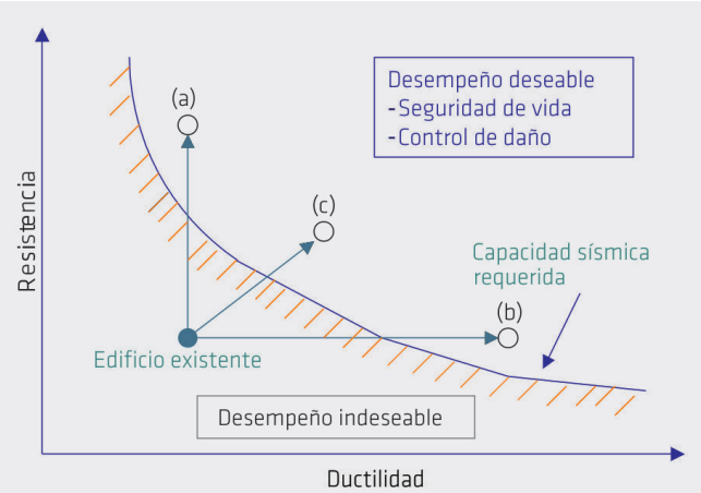
Figura 2. Estrategias de intervención sísmica y posibles niveles de desempeño [1].
