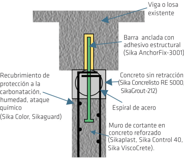
Figura 4. Detalle de la conexión en la parte superior de una pantalla en concreto reforzado
