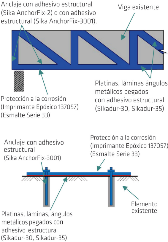
Figura 14. Reforzamiento con platinas, láminas, ángulos de acero
