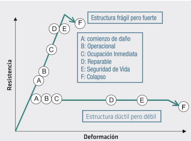
Figura 3. Posibles localizaciones de los niveles de desempeño para diferentes estructuras [3].
