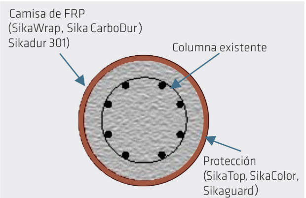
Figura 26. Encamisado o envoltura con laminas o platinas CFRP, GFRP, AFRP en reforzamiento de columnas.
