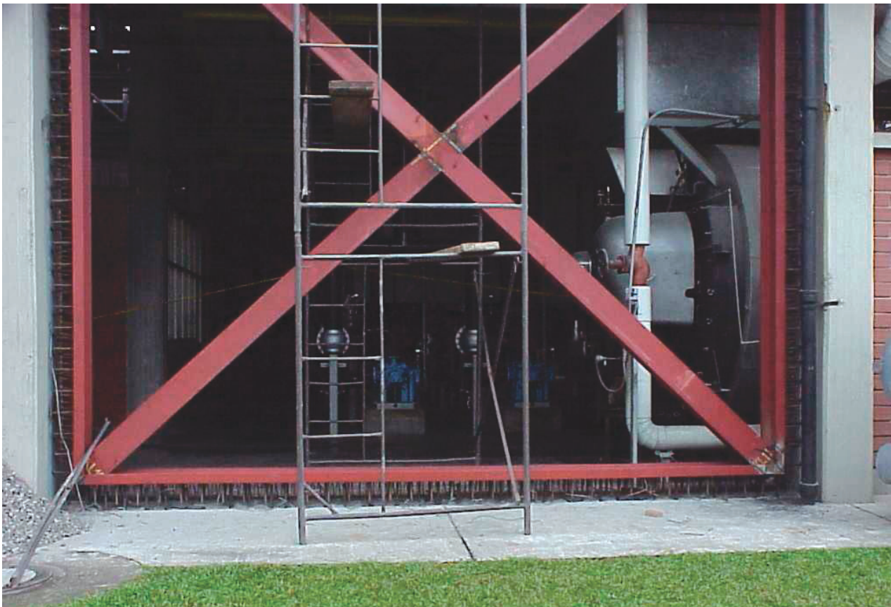
Arriostramiento metálico con conexión indirecta en edificio industrial
