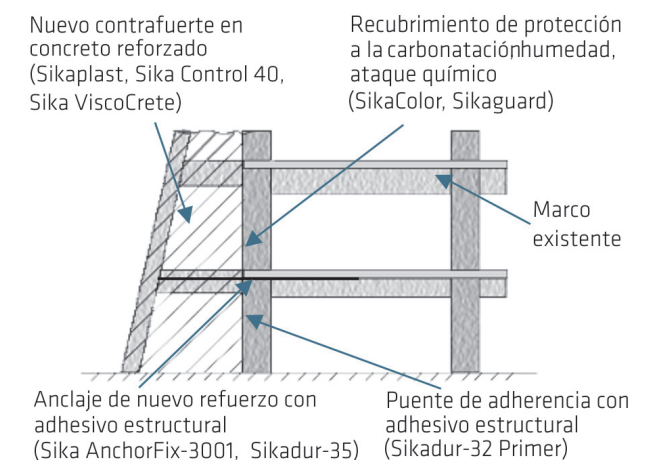
Figura 10. Contrafuerte de concreto reforzado adosado a la estructura existente.
