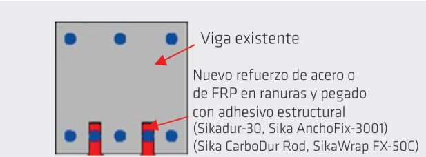
Figura 15. Instalación de varillas de acero o de FRP en ranuras en el reforzamiento de una viga.
