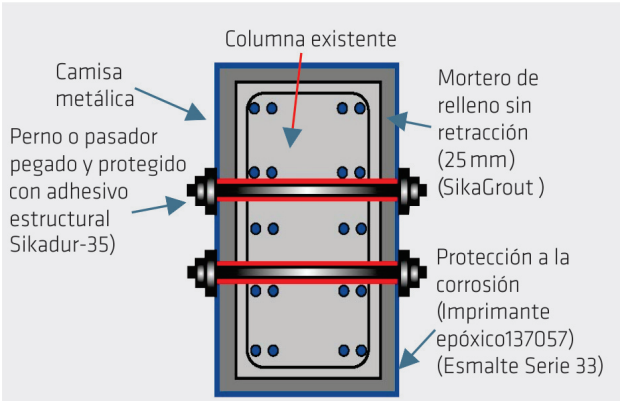
Figura 23. Columna con traslapeo inadecuado reforzado mediante camisa de acero y pernos de anclaje o pasadores adheridos y con concreto o mortero de relleno.
