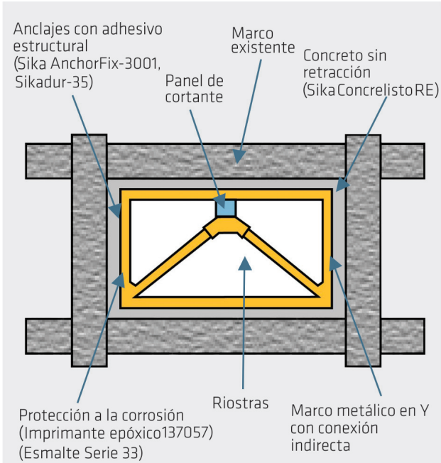
Figura 27. Reforzamiento sísmico con riostras dúctiles de acero con conexión indirecta.
