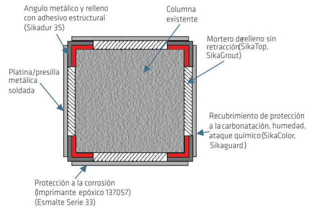
Figura 25. Enchaquetado con ángulos y platinas metálicas.
