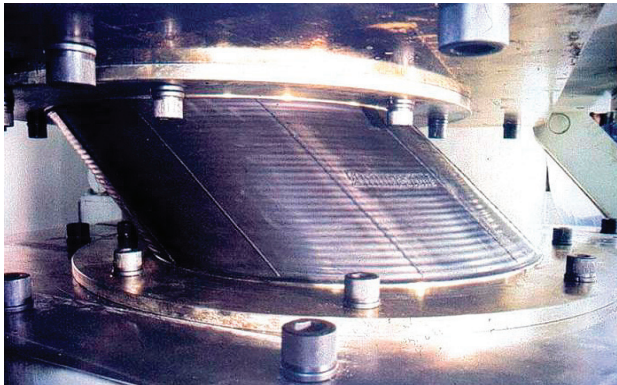
Prueba de aislador (Bridgestone)
