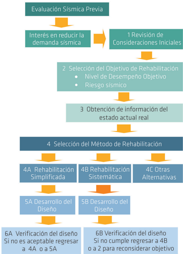
Figura 1. Proceso de rehabilitación según FEMA 356 [4].
