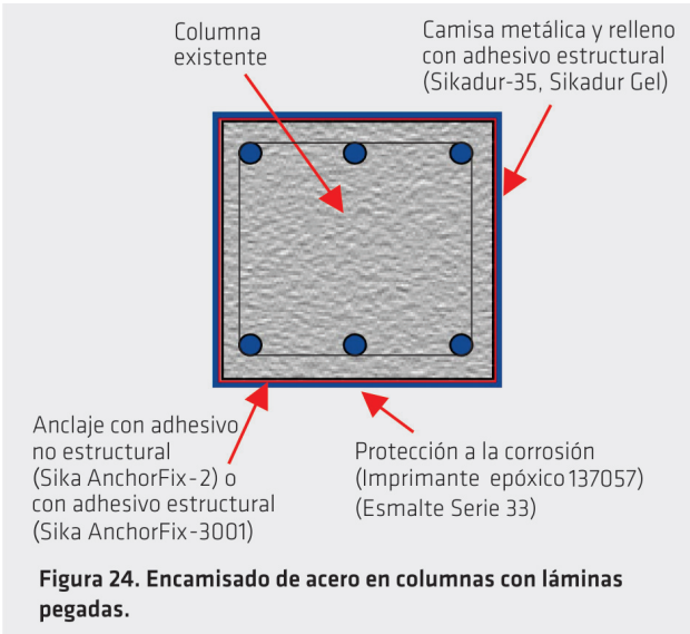
Figura 24. Encamisado de acero en columnas con láminas pegadas.
