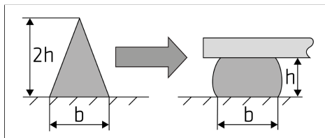
Figura 1: Cordón de adhesivo recomendado
