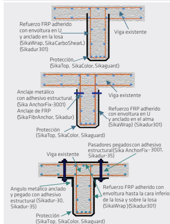
Figura 18. Instalación de platinas o laminas CFRP o GFRP ancladas en el reforzamiento de una viga a cortante.
