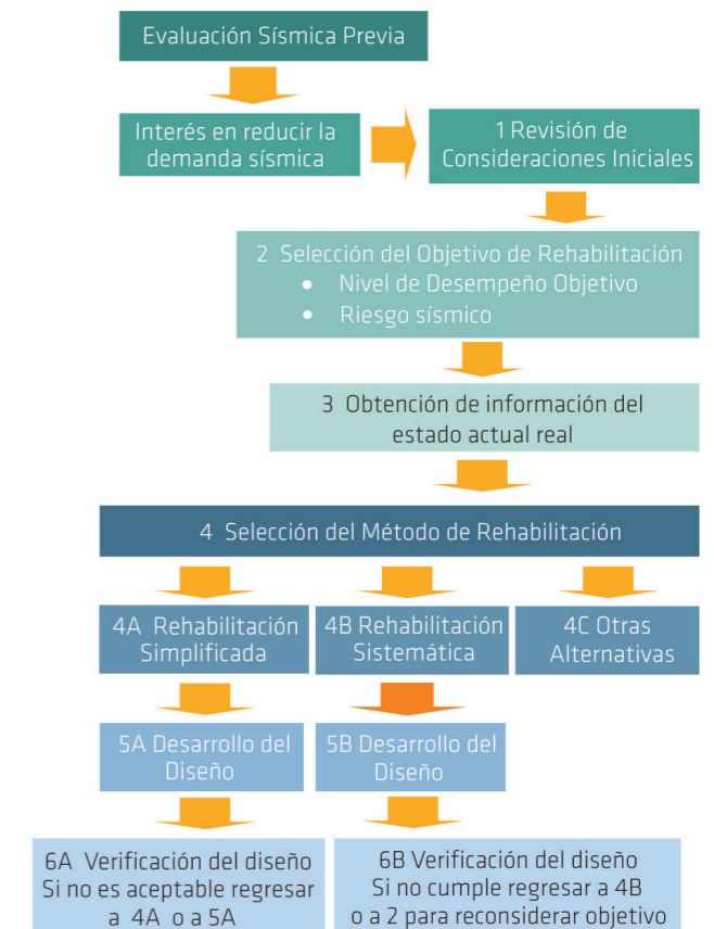
Figura 1. Proceso de rehabilitación según FEMA 356 [4].
