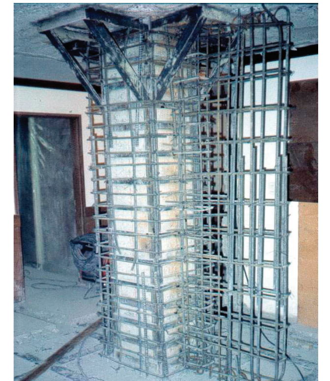
Encamisado y adición de muro lateral en concreto reforzado de columna en edificio comercial
