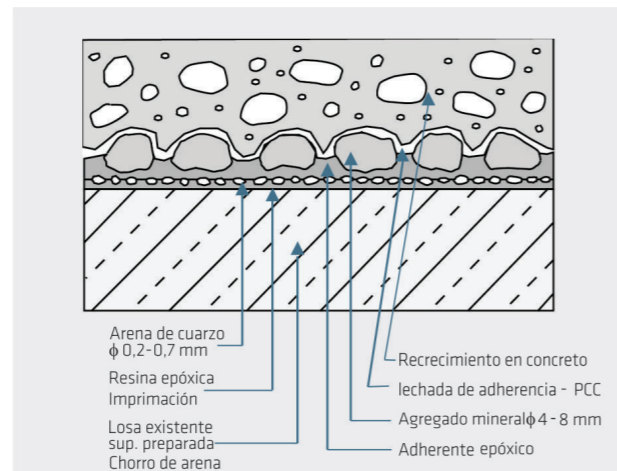
Figura 12. Engrosamiento superior con concreto y sistema de adherencia con adhesivos y agregados para aumento de la capacidad portante de una losa de concreto [9].
